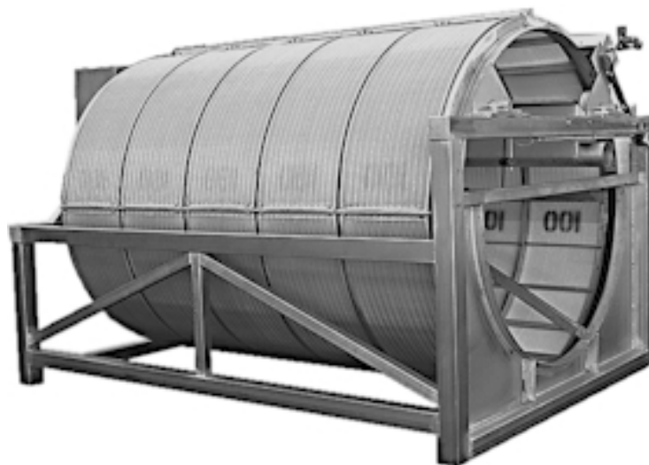
Figura 5: Filtro mecânico tipo tambor usado em sistema de recirculação de água
